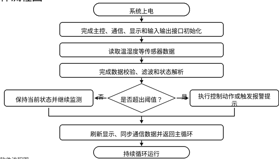
图2 软件流程图
