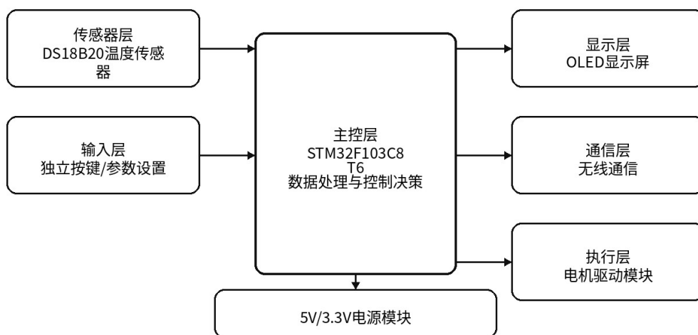
图1 系统框架图
