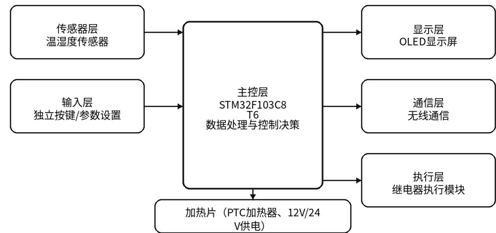
图1 系统框架图
